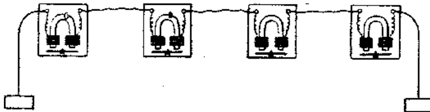
Telefonische Leitung Alexander Graham Bells Sprechtelegraph.
