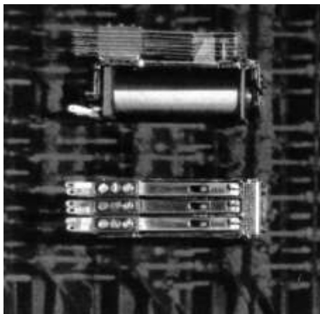
Das Relais 46
