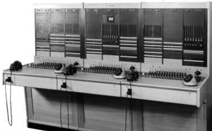
III S anreihbare Bedienplätze
