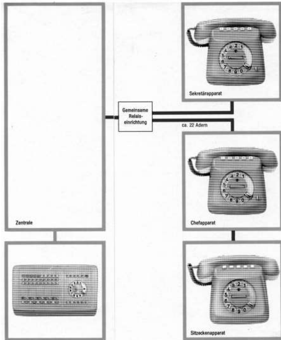
Pikkoloanlagen der Lieferserie E 1 und E 2
