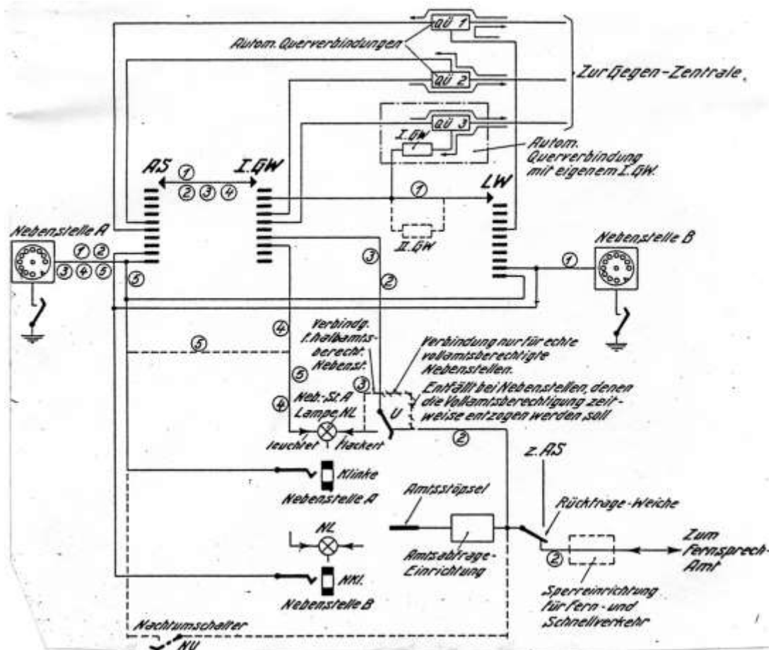
Prinzip-Darstellung eines Verbindungsaufbaues
