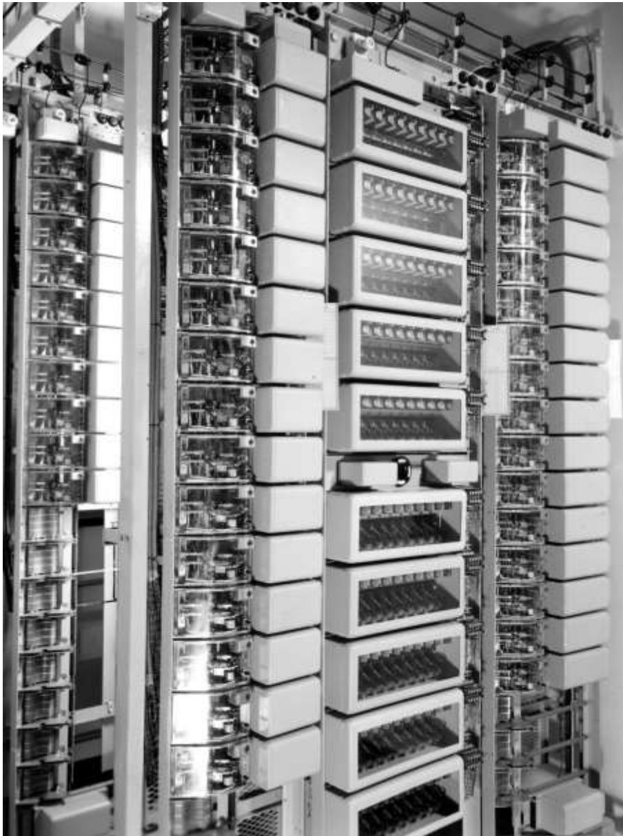
Teilansicht des Wählerteiles mit Gruppen-, Vor- und Leitungswähler zu einer III S Anlage mit 200 Teilnehmern
