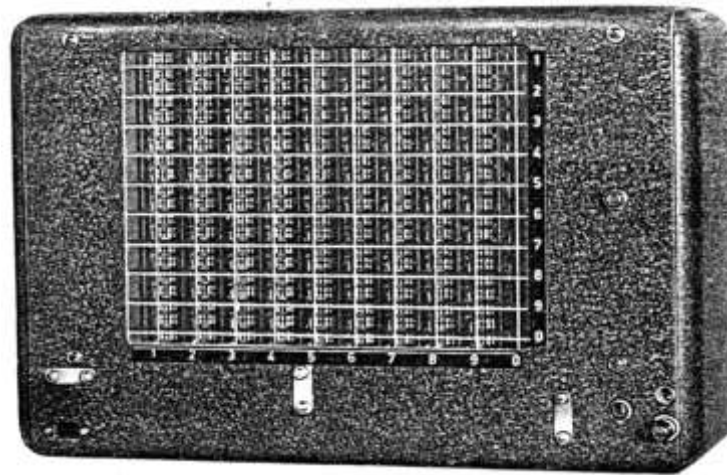
TN Edelmetallkontaktwähler (Kreuzschienenwähler) mit Schutzkappe, 100 teilig, 4 adrige Durchschaltung
