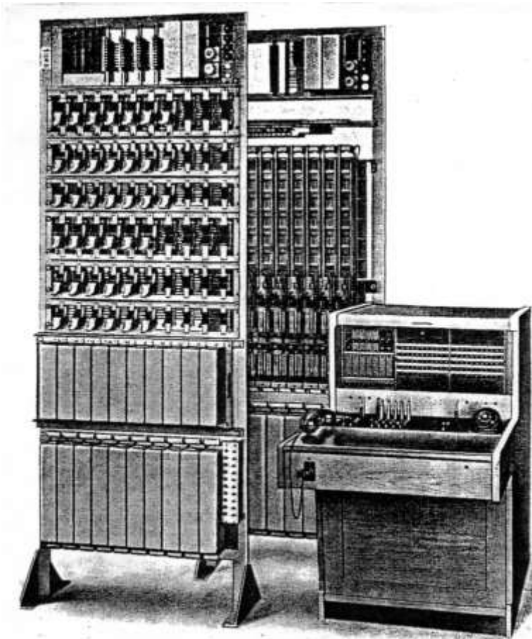
II G Rekordzentrale, 10 Amt 100 Nebenstellen
