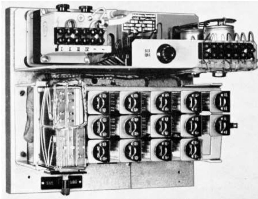
Zwischenstellenumschalter mit abgenommener Schutzkappe
