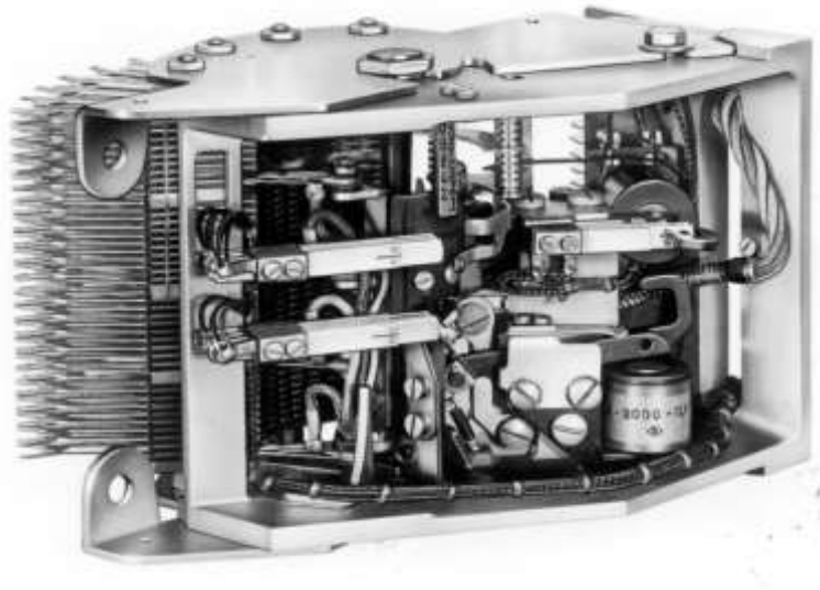
TN Viereckwähler mit Wälzankerantrieb
