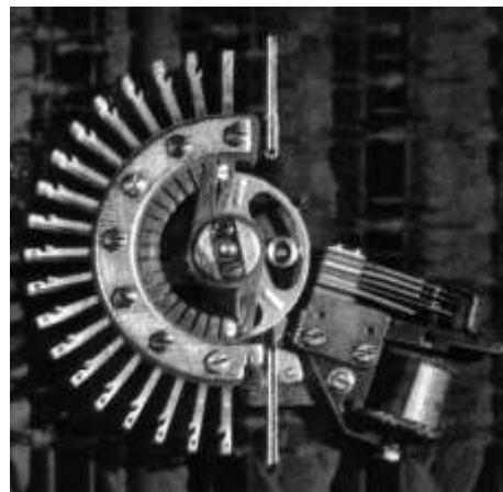
Drehwähler mit Wälzankerantrieb
