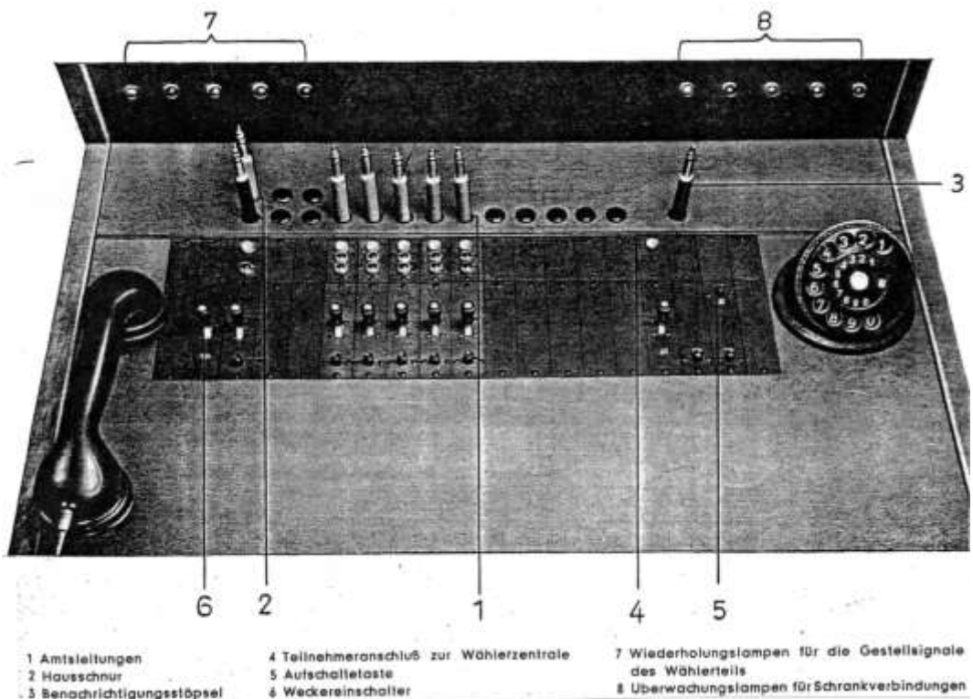
Abfrage- und Bedienungsplatz einer REKORD-Zentrale (Einschnurssystem)
