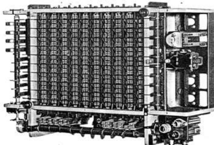
TN Kreuzschienenwähler ohne Schutzkappe
