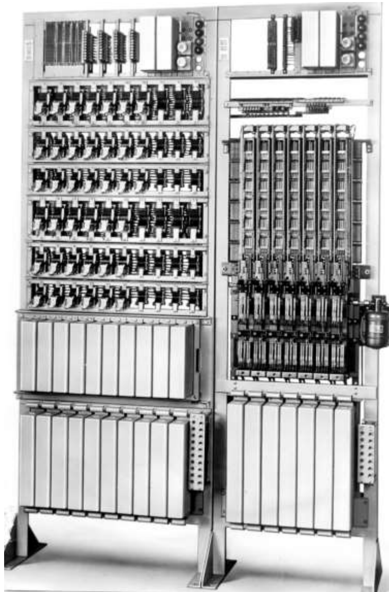
Rekordzentrale IIG - S
