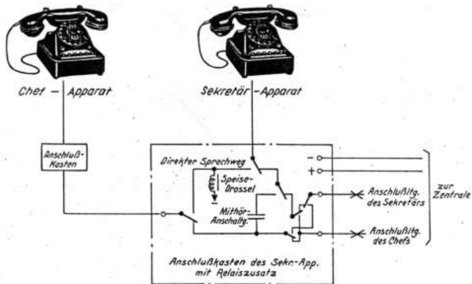
Prinzip der Pikkoloanlage
