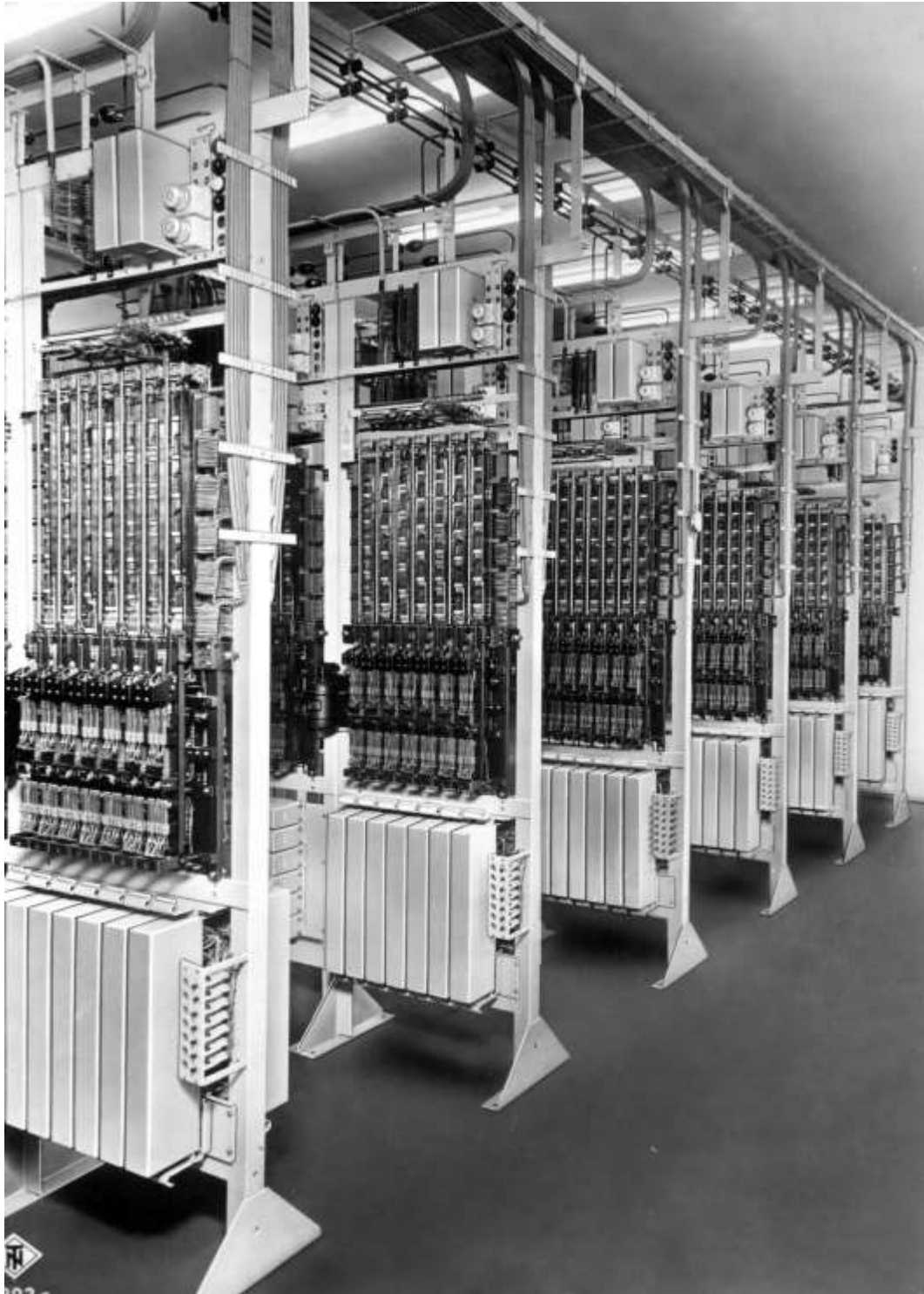
6 Hunderter Gruppen einer Fallwähleranlage IIIW
