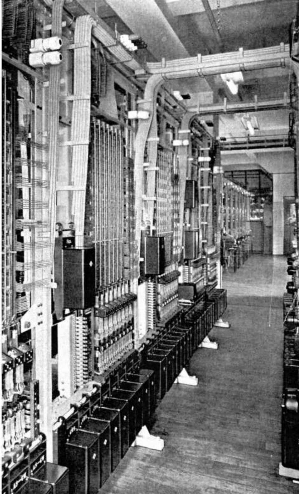
Wählersaal, Teilansicht (Henkelwerke Düsseldorf)
