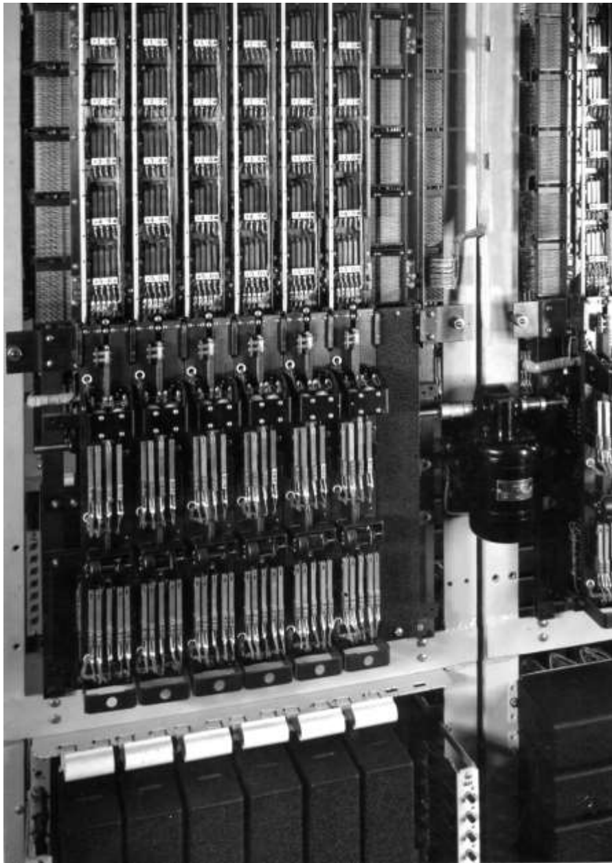
1950 Teilansicht der Fallwähler, Anrufer-Leitungswähler
