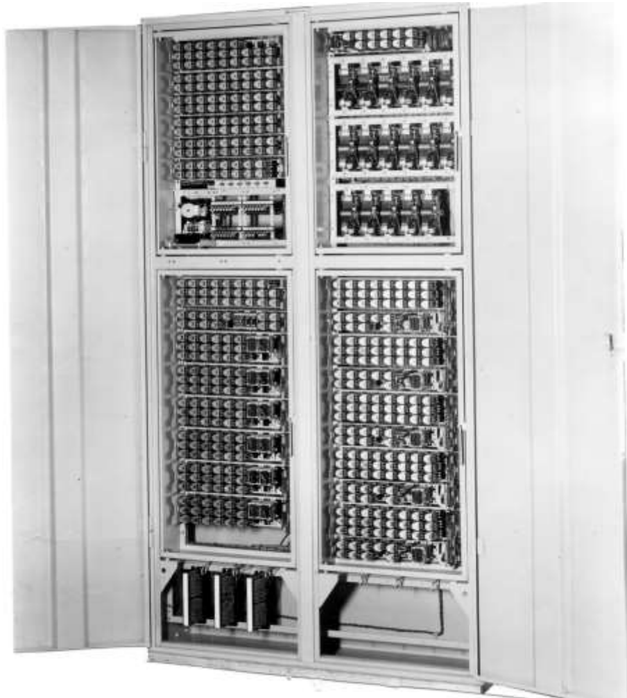
Geöffneten Schrank der Anlage IIE
