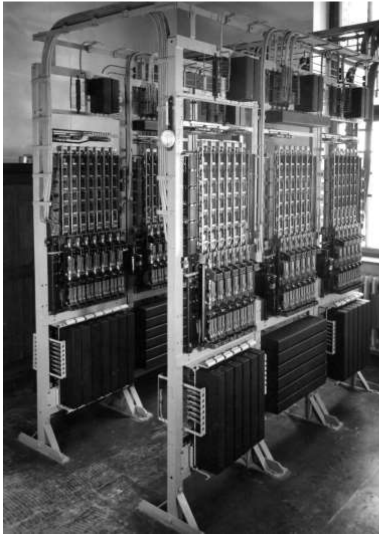
1950 Fallwähler für 200 Teilnehmer
