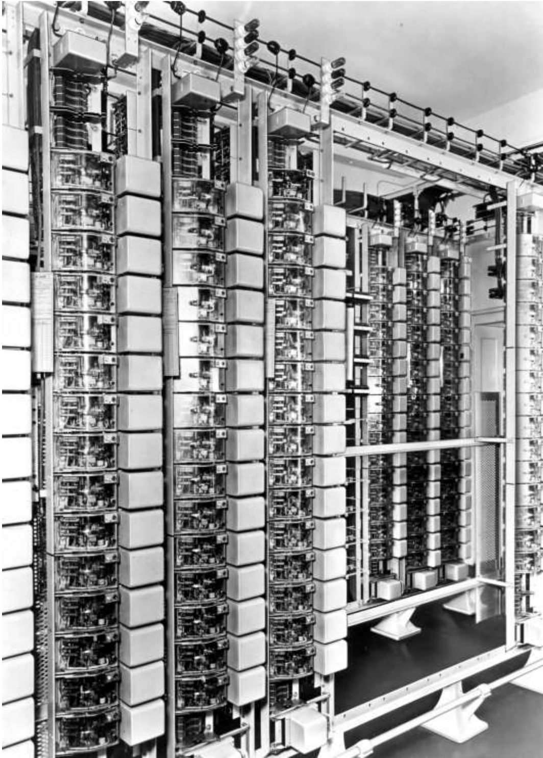
Teilansicht einer Viereckwähleranlage IIIW
