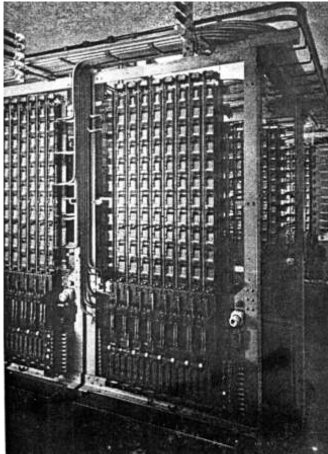
Fallwählerzentrale (Harburger Gummiwarenfabrik Phönix)
